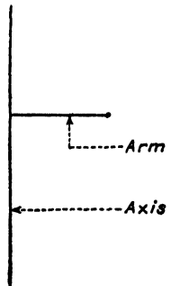
FIG. 1.—Cyclic axis.
